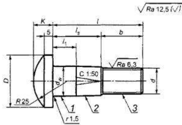
Рисунок 2 - Болты конические высокопрочные с полукруглой головкой
