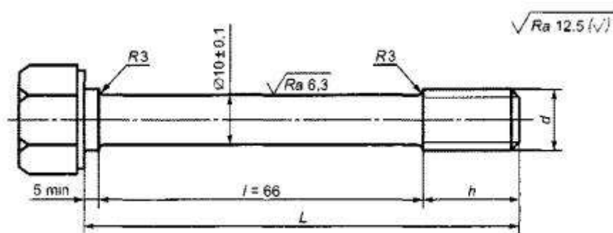
Рисунок 7 - Обработанный образец для испытания на растяжение
