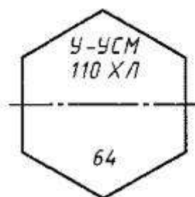
Рисунок 6 - Маркировка гаек
